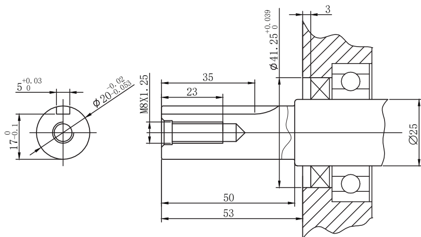
Obr. 1, výkres hriadeľa motora Heron® 8896670
