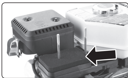
Obr. 7, ilustračný obrázok umiestnenia vzduchového filtra
