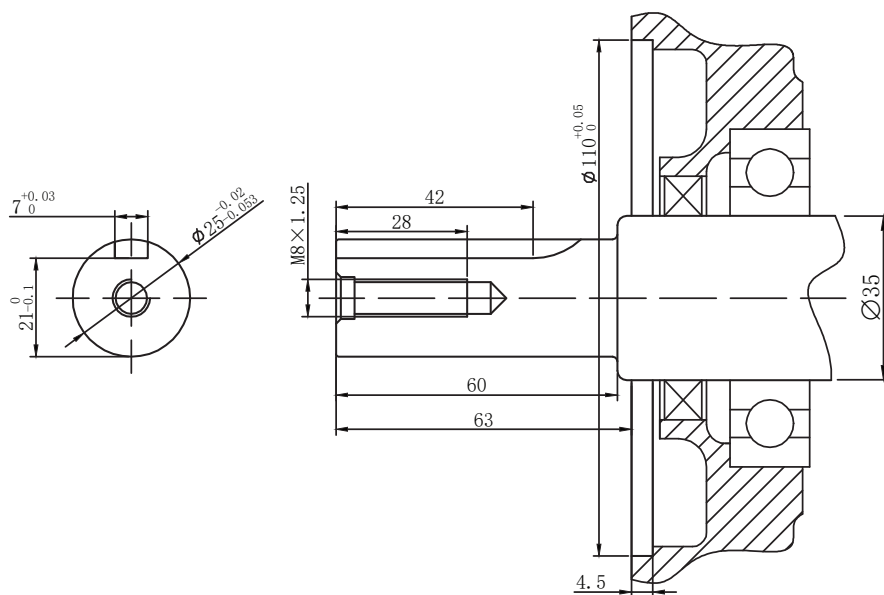
Obr. 2, výkres hriadeľa motora Heron® 8896670
