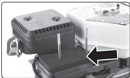
Obr.7, ilustrační obrázek umístění vzduchového filtru
