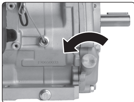
Obr.4, uzávěr olejové vany pro nalití oleje
